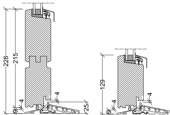
Alubundstykke Indadgående dør Lodret snit
