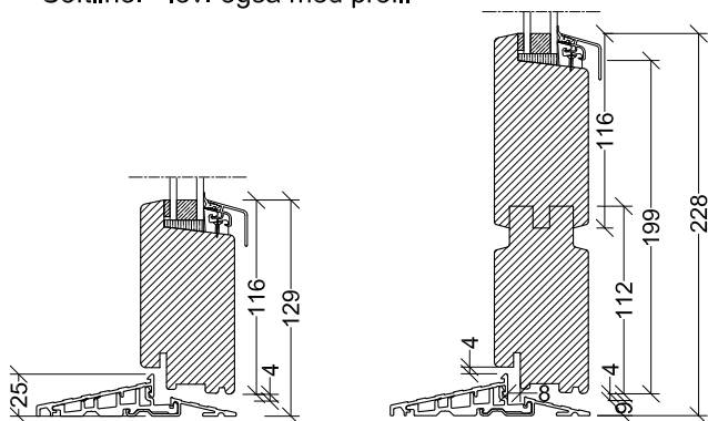
Alubundstykke Udadgående dør Lodret snit
