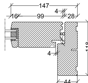
Indadgående dør Vandret snit
