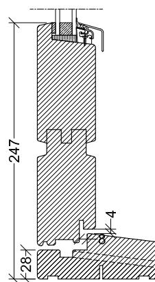
Indadgående dør Lodret snit
