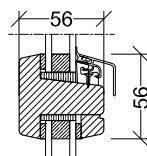
Smal sprosse Lodret snit
