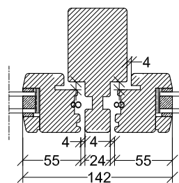
Sidehængt / topstyret ramme Vandret snit
