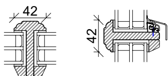
42 mm sprosser
