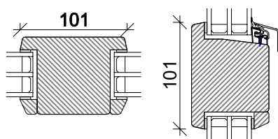
101 mm sprosser
