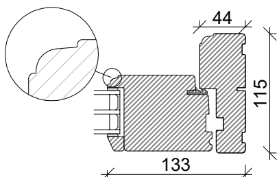
Midt dobbeltdør M/ profil udadgående
