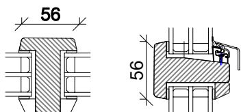
56 mm sprosser
