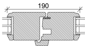
Midt dobbeltdør M/ profil udadgående
