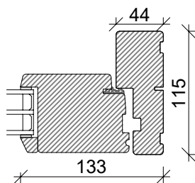
Sidekarm
