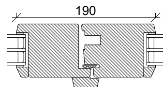
Midt dobbeltdør Indadgående
