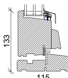
Bundkarm indadgående
