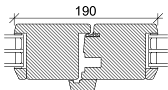
Midt dobbeltdør Udadgående
